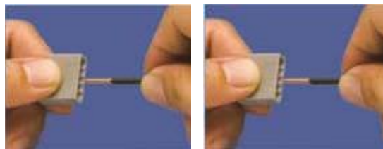
2- Kablo sıralamalarından emin olduktan sonra tüm kabloları sokete itiniz.
