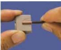
1- Kablo Boyu 11mm olacak şekilde açınız.
